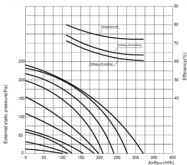
KE250H Entalpica
