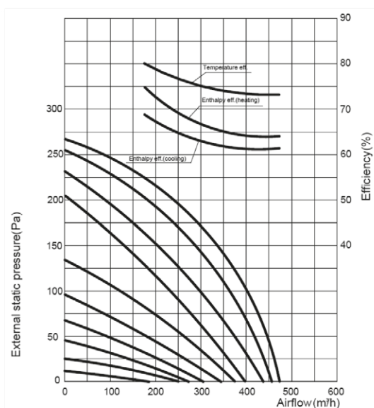
KE350H Entalpica
