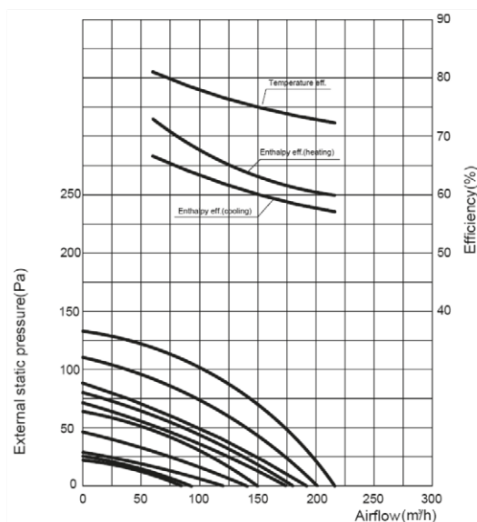
KE150H Entalpica
