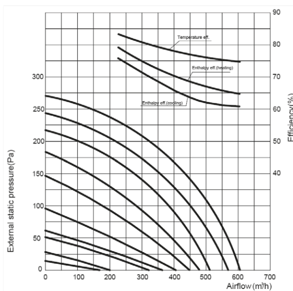
KE500H Entalpica
