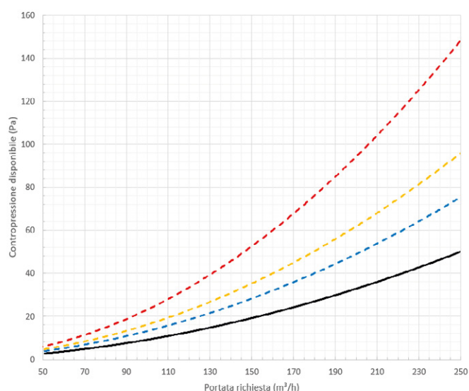
Caratteristica VENTILATORE ESPULSIONE
