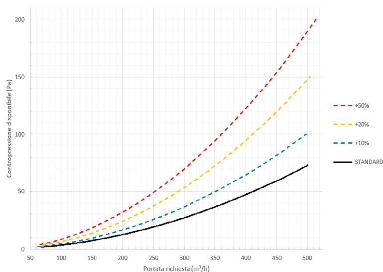
Caratteristica VENTILATORE TOTALE
